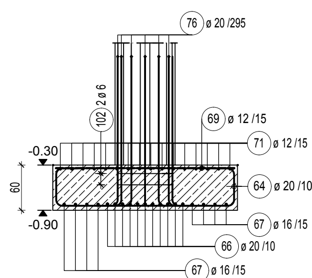
OC-6
