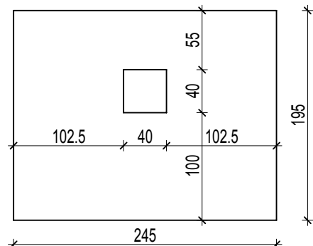
OC-2 (szalunek)
